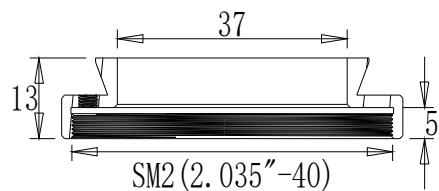
截面 A-A
