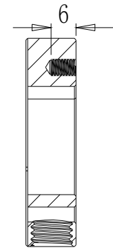
截面 A-A
