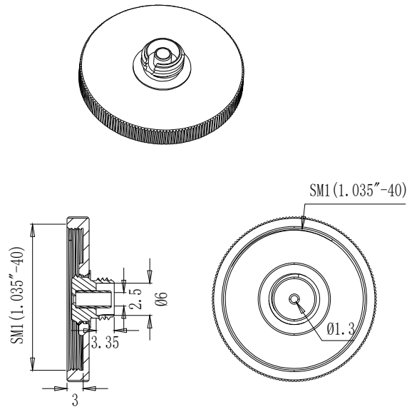
截面 A-A
