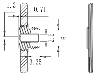
截面 A-A
