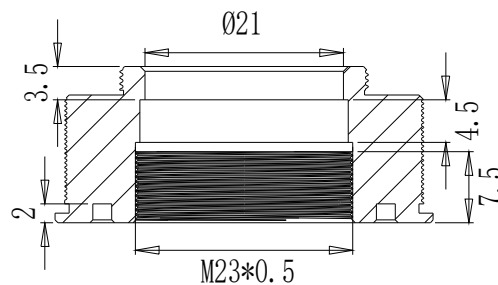
截面 A-A
