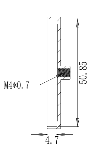
截面 A-A
