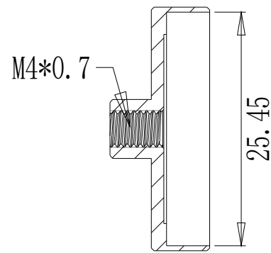
截面 A-A
