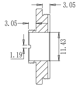
截面 A-A
