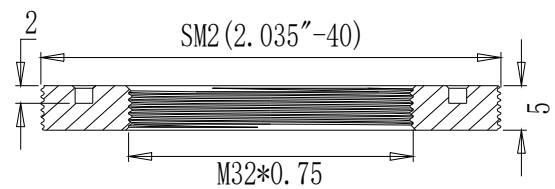
截面 A-A
