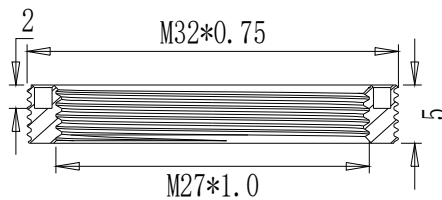
截面 A-A
