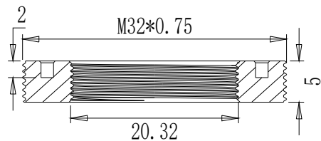
截面 A-A
