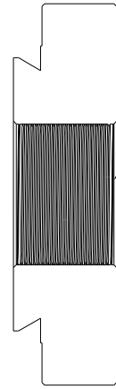
截面 A-A
