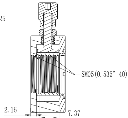
截面 A-A
