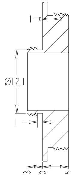
截面 A-A
