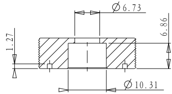
截面 A-A
