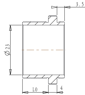
截面 A-A
