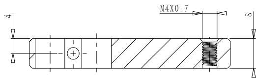
截面 A-A
