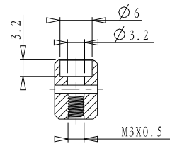
截面 B-B
