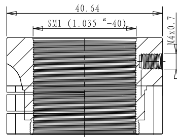
截面 A-A
