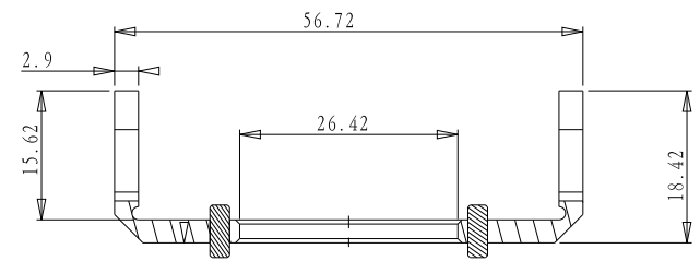
截面 A-A
