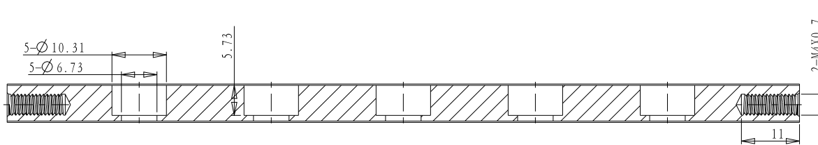
截面 A-A
