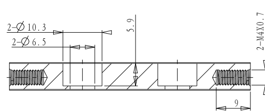
截面 A-A
