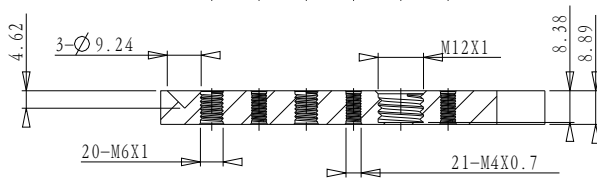
截面 B-B
