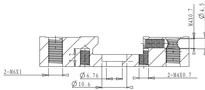
截面 A-A
