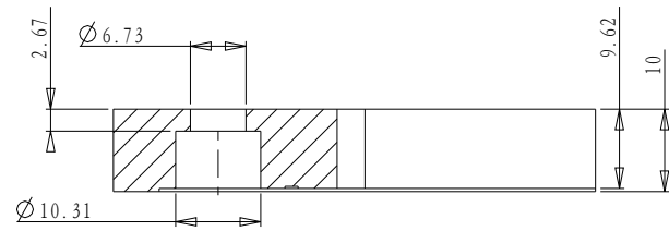
截面 A-A
