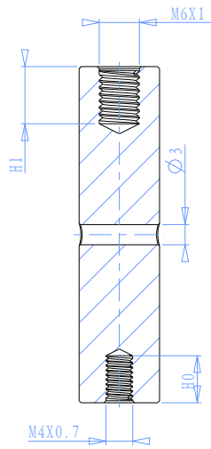
截面 A-A
