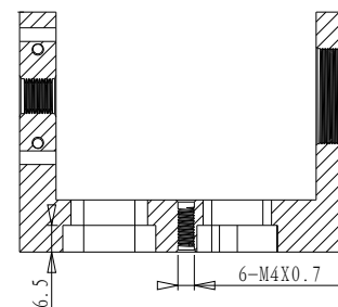
截面 E-E
