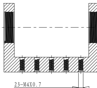
截面 D-D
