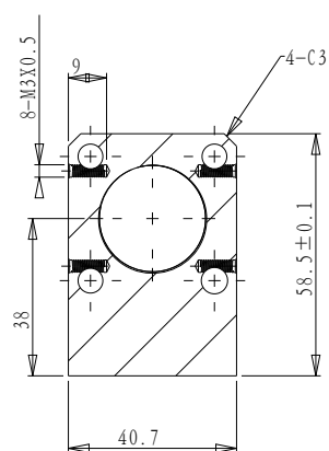
截面 B-B
