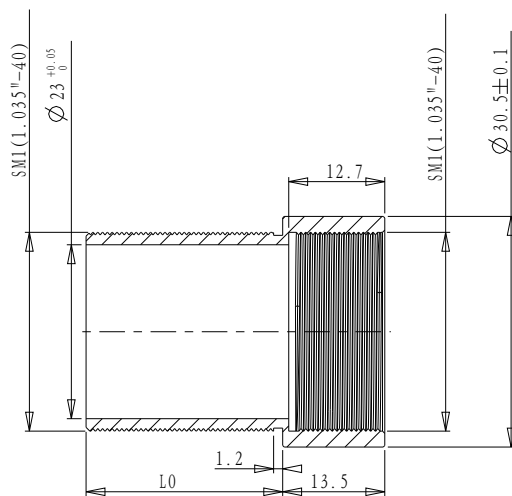
截面 A-A
