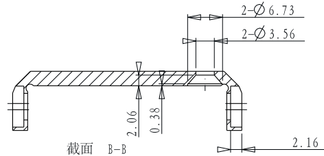
截面 B-B
