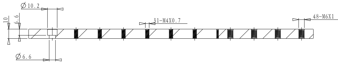
截面 A-A
