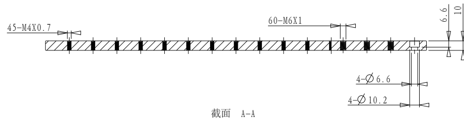
截面 A-A
