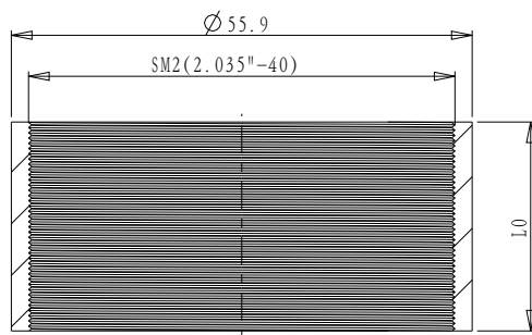
截面 A-A
