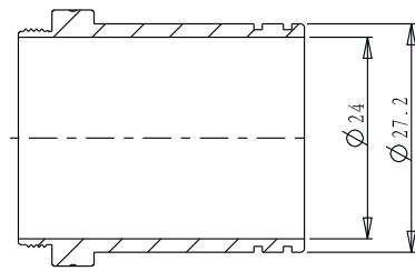
截面 A-A
