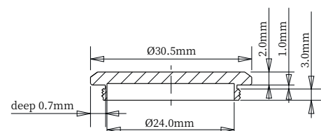
截面 A-A
