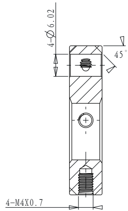
截面 B-B
