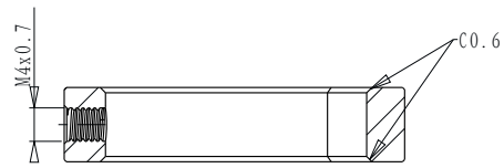
截面 A-A
