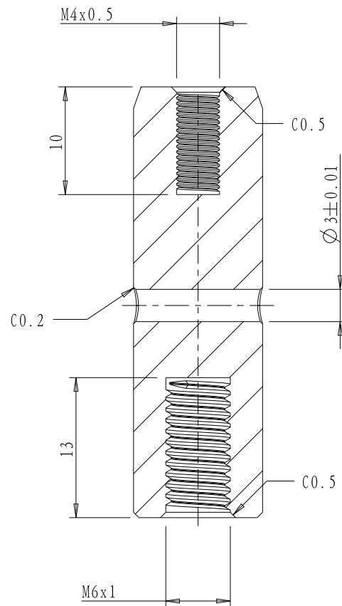
截面 A-A
