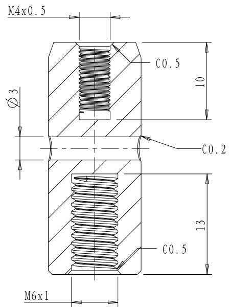
截面 A-A
