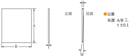
外型图 >
