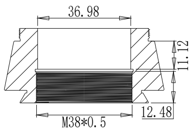
截面 A-A
