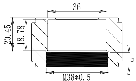
截面 A-A
