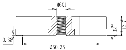
截面 A-A
