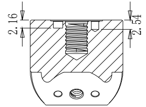
截面 B-B
