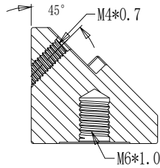
截面 A-A
