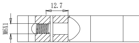
截面 A-A
