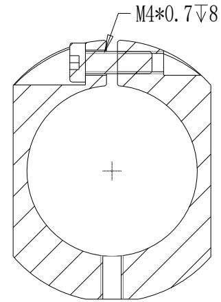
截面 A-A
