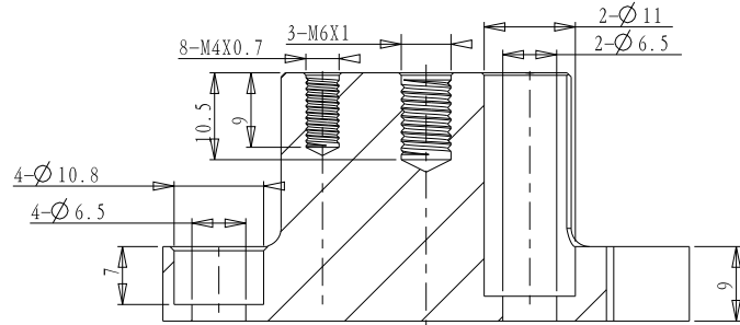
截面 A-A
