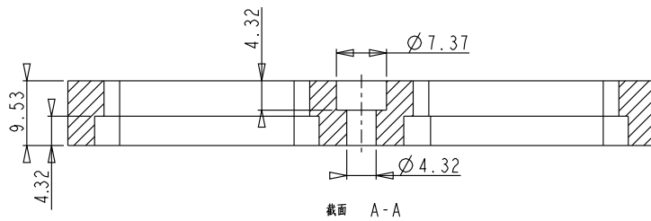
截面 A-A
