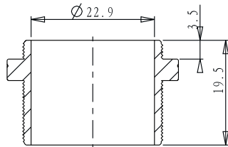
截面 A-A
