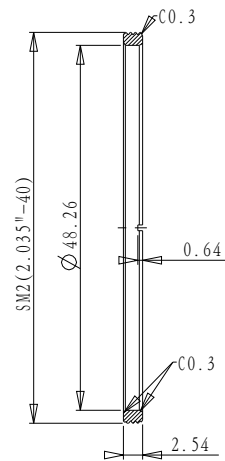
截面 A-A
