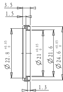
截面 A-A
