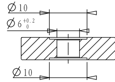
截面 A-A
