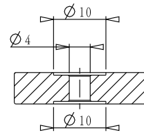
截面 A-A
